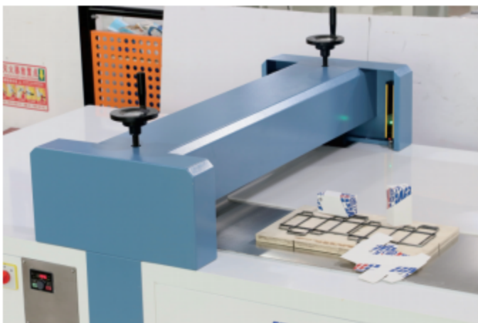
上下滚筒，压力均匀 Uniform Pressure
