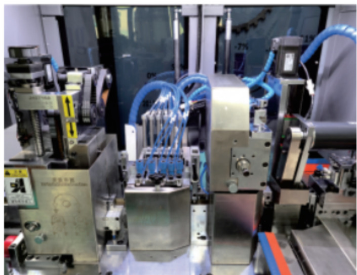
多组磨边打点、多功能 冲切、沉孔 Multi Functions Punch, Countersunk Hole, Nick
